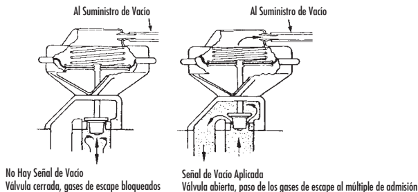
FIGURA 7: OPERACIÓN DE LA VÁLVULA DE RECIRCULACIÓN DE LOS GASES DE ESCAPE
