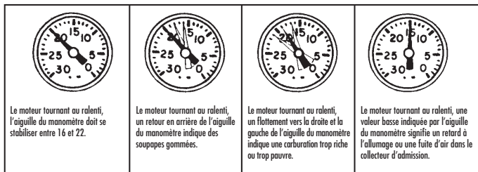
FIGURE 5: INDICATIONS DU MANOMÈTRE À VIDE
