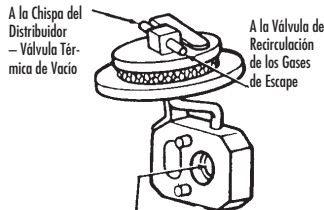
Expuesta a la Presión de los Gases de Escape
