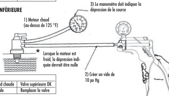
FIGURE 15: CONTRÔLE DE LA VALVE DE COMMUTATION DE DÉPRESSION À QUATRE ORIFICES
