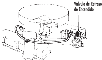
FIGURA 12: VÁLVULA DE RETRASO DE ENCENDIDO TÍPICA
