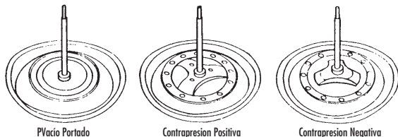
FIGURA 8: DIAFRAGMAS DE RECIRCULACIÓN DE LOS GASES DE ESCAPE FABRICADOS POR GM
