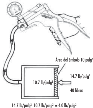
FIGURA 1: EL VACÍO Y LA PRESIÓN ATMOSFÉRICA
