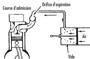
FIGURE 2: LE MOTEUR COMME SOURCE DE VIDE
